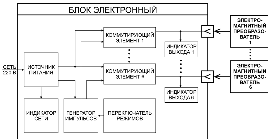
Рис. 1 Структурная схема импульсатора ЭИ-102-6
